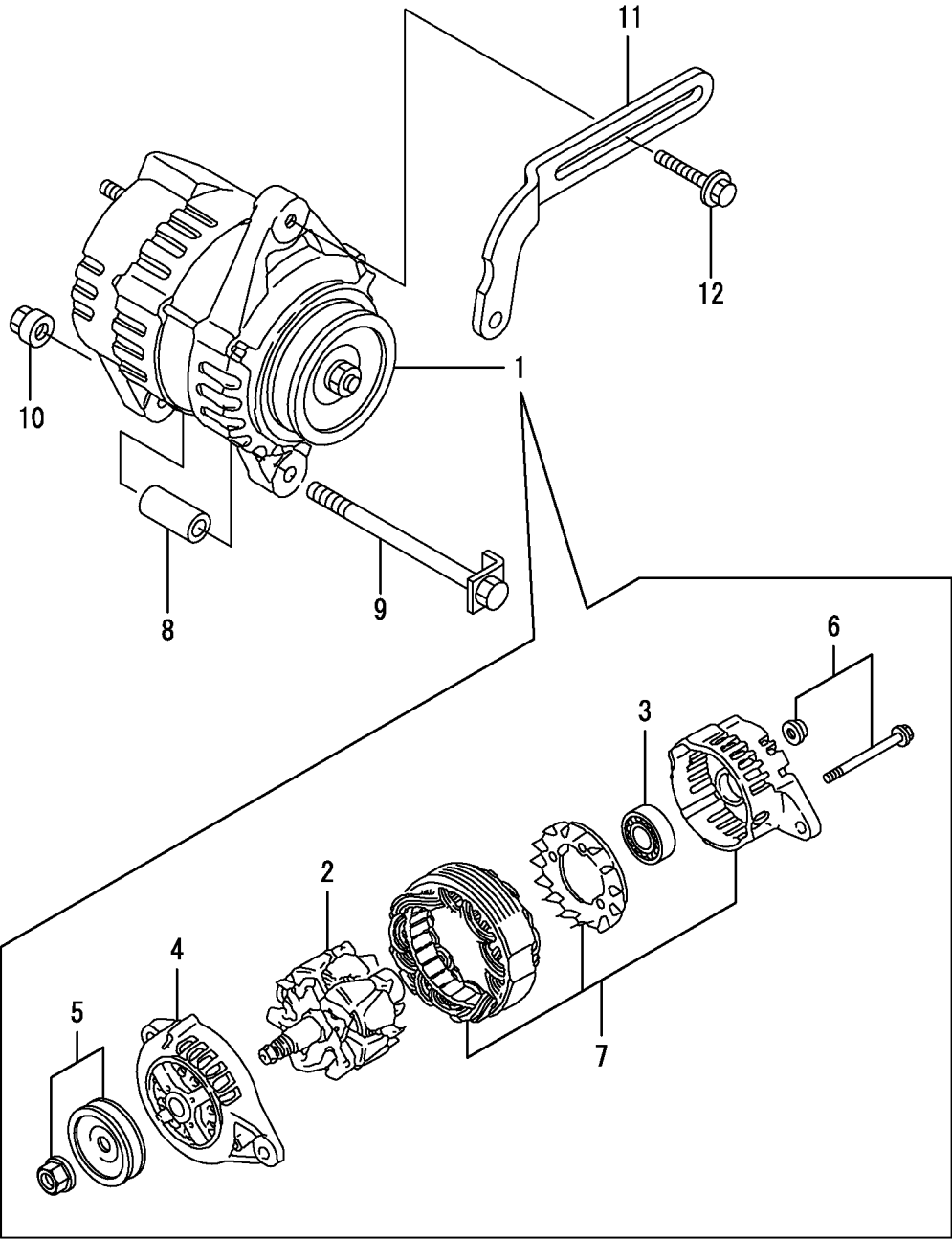
Fig.16. GENERATOR
